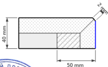
ВИД ЛИЦЕВОГО ПРОФИЛЯ
