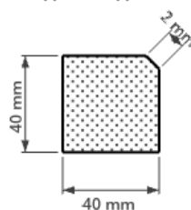
ВИД НАКЛАДНОГО БОРТА
